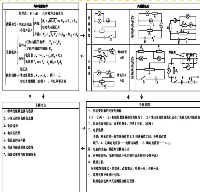
仵希洁 (12.1班) 同学作品——伏安法测电阻
